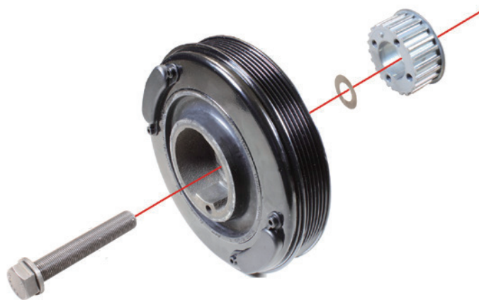
画像 1：クランクシャフト振動ダンパーとクランクシャフトのセントラルボルト、ダイヤモンドワッシャー
